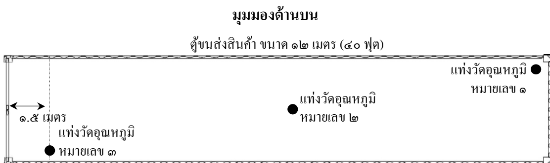
ภาพที่ ๑ ตำแหน่งการวางแท่งวัดอุณหภูมิผลไม้ภายในตู้ขนส่งสินค้าสำหรับการกำจัดศัตรูพืชด้วยความเย็นในระหว่างขนส่ง
